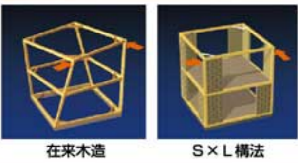
在来木造 S×L構法
